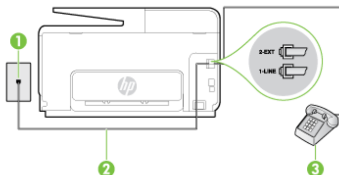
Figure B-4 Vue arrière de l'imprimante
