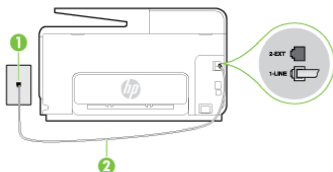
Figure B-1 Vue arrière de l'imprimante
