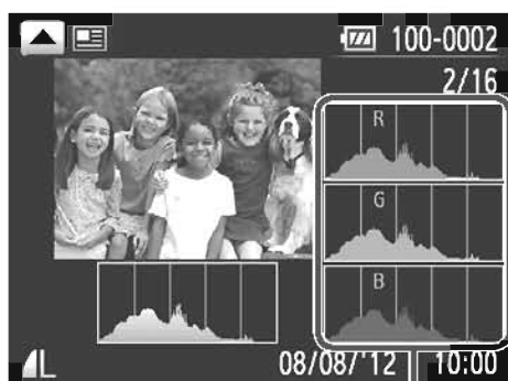
Histogramme RVB
