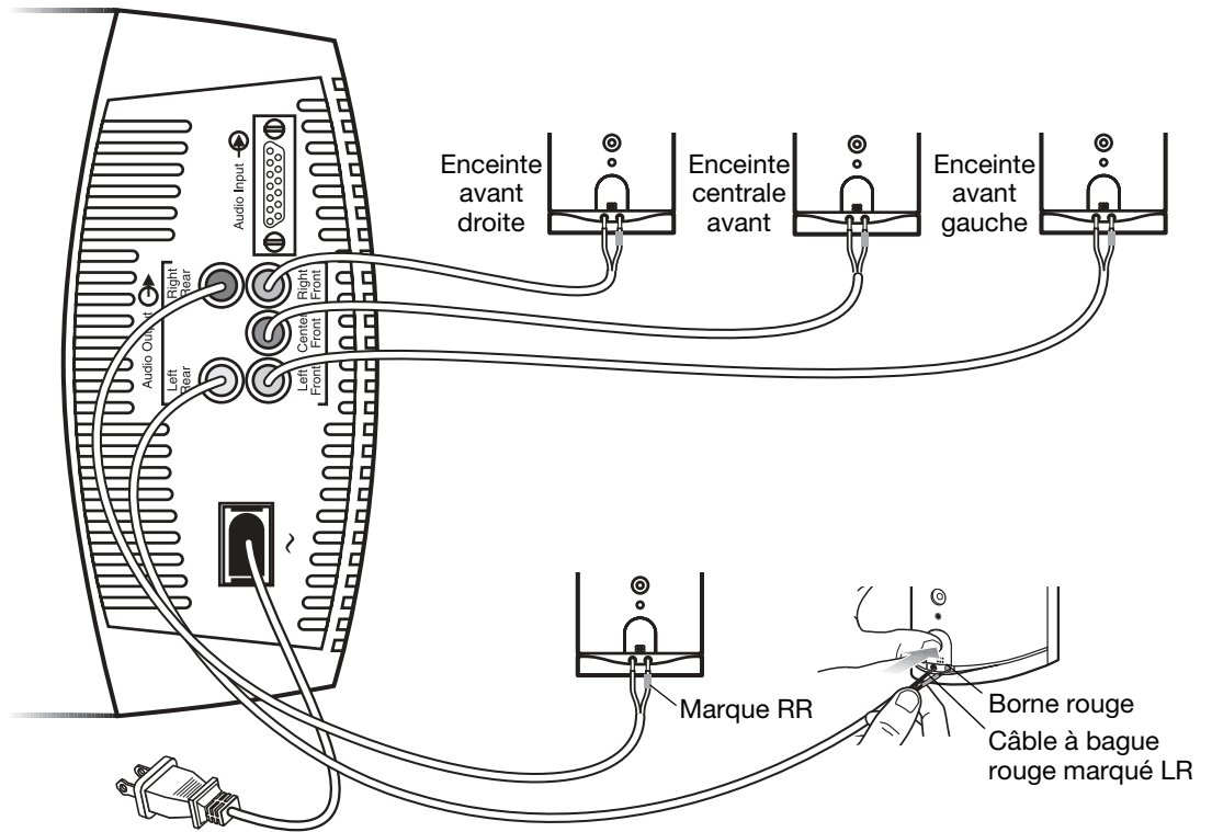
Module Acoustimass® 10
