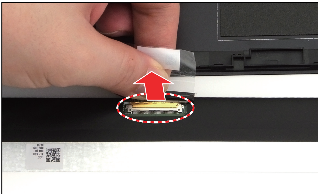
Figure 1-46. Débrancher le câble eDP
