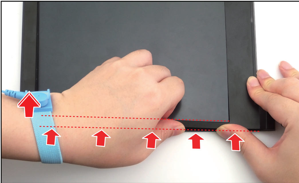
Figure 1-39. Retirer l'encadrement LCD (5 sur 8)
