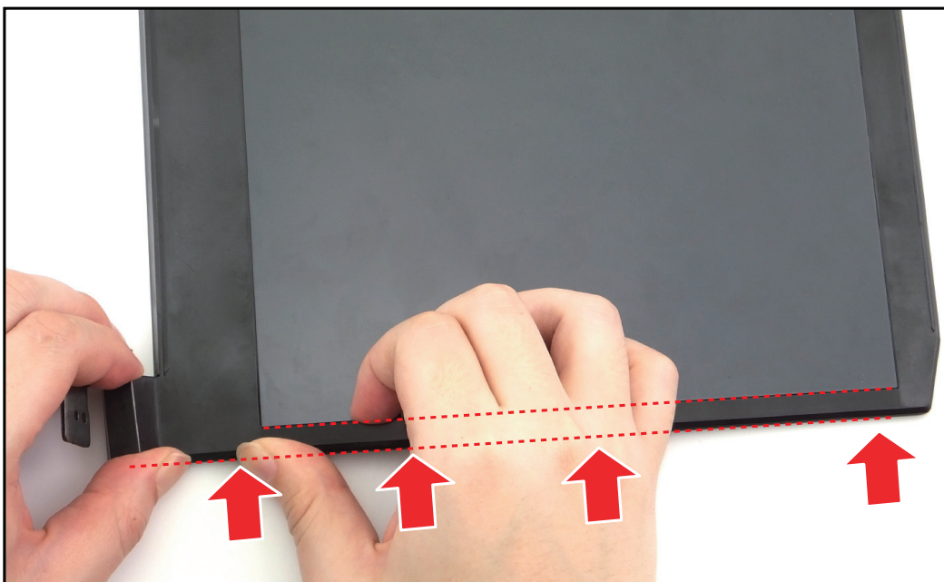
Figure 1-36. Retirer l'encadrement LCD (2 sur 8)
