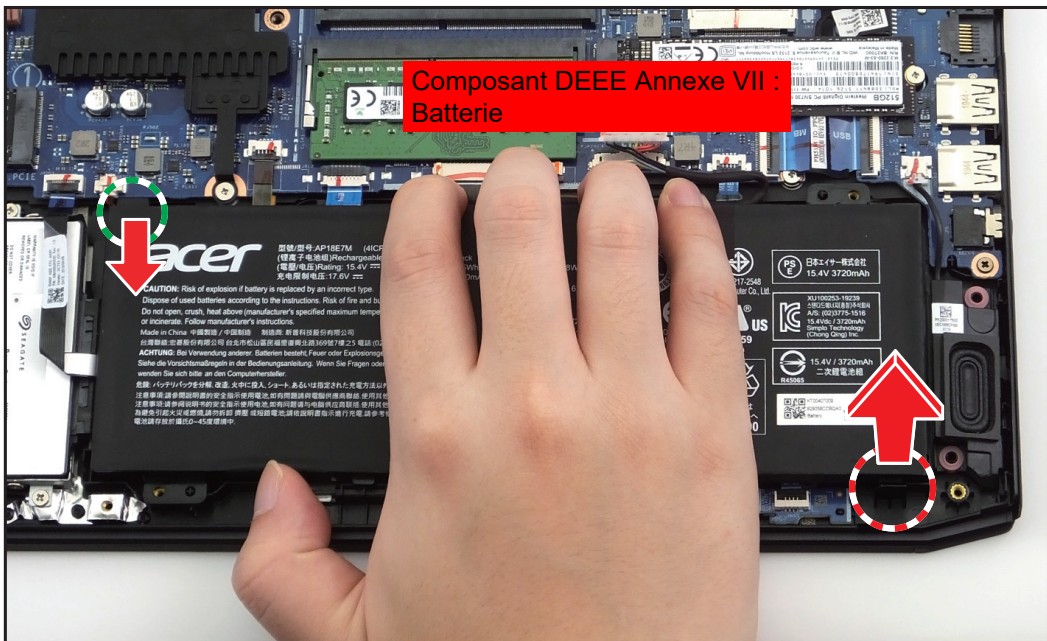
Figure 1-7. Retirer la batterie
