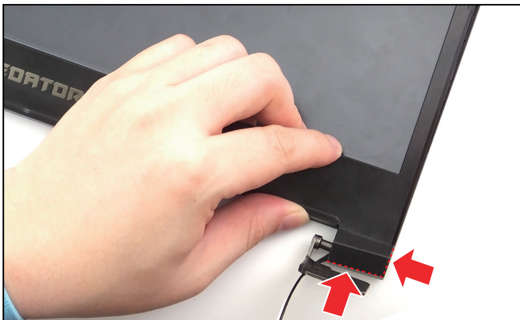
Figure 1-42. Retirer l'encadrement LCD (8 sur 8)
