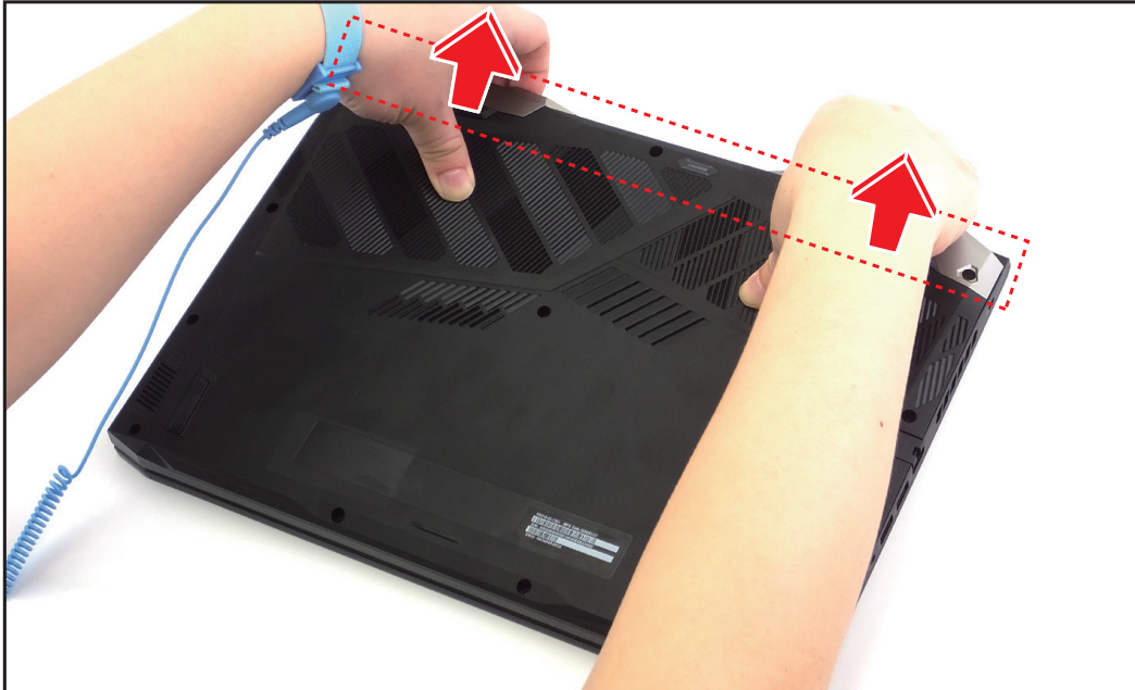
Figure 1-3. Libérer le boîtier inférieur (1 sur 2)
