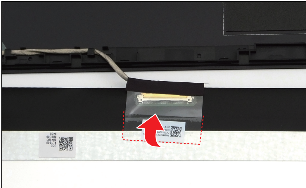
Figure 1-45. Détacher le Mylar
