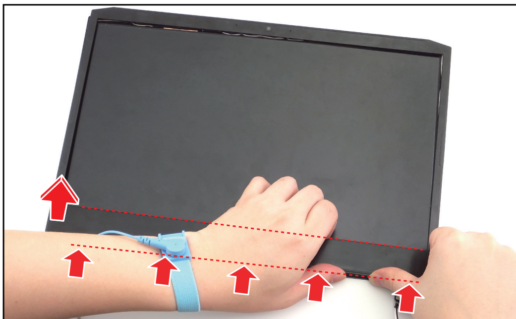
Figure 1-41. Retirer l'encadrement LCD (7 sur 8)
