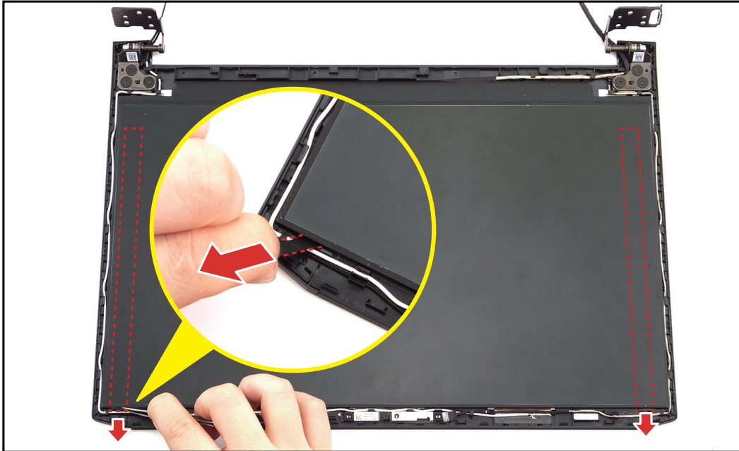
Figure 1-43. Détacher les rubans de montage double face
