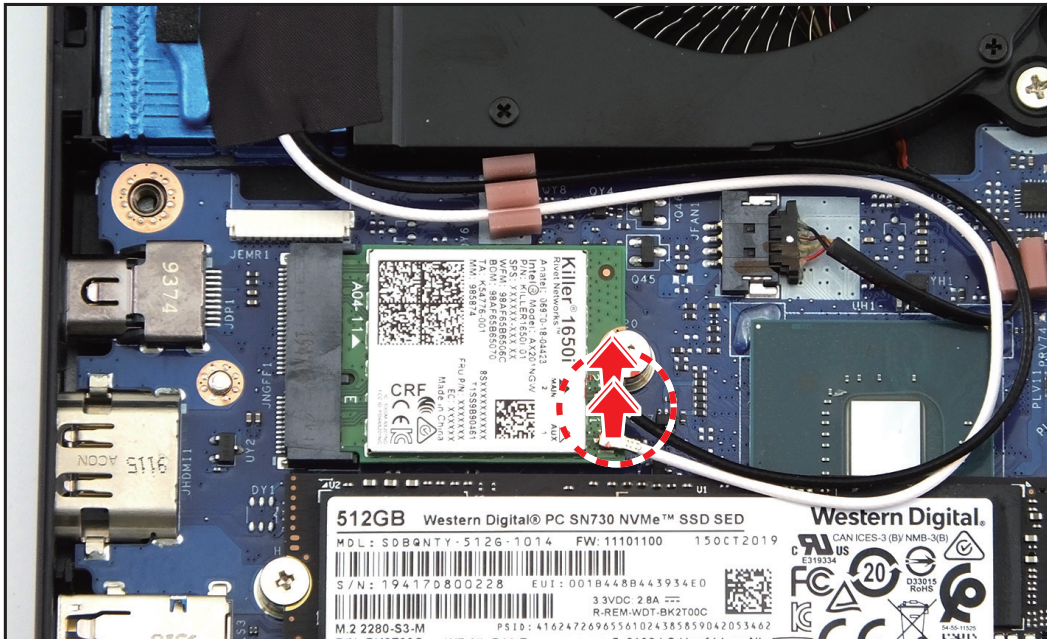
Figure 1-8. Débrancher les câbles de l'antenne WLAN
