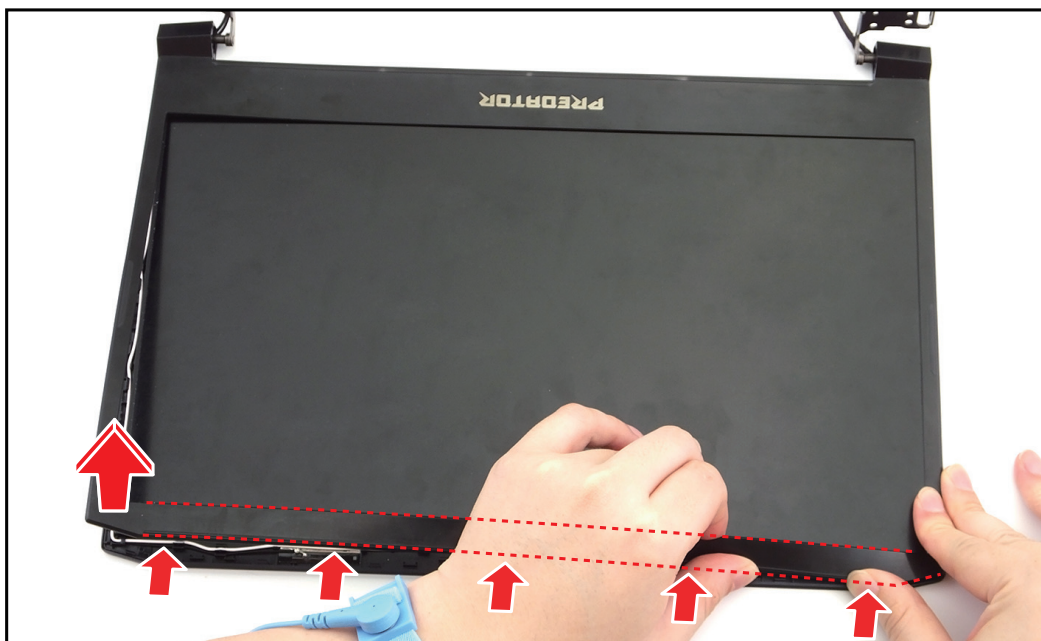
Figure 1-38. Retirer l'encadrement LCD (4 sur 8)
