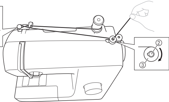
① Disque de pré-tension ② Axe du dévidoir ③ Canette
