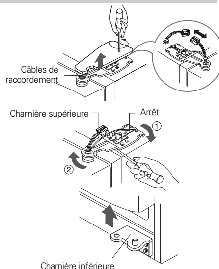
Charnière inférieure
