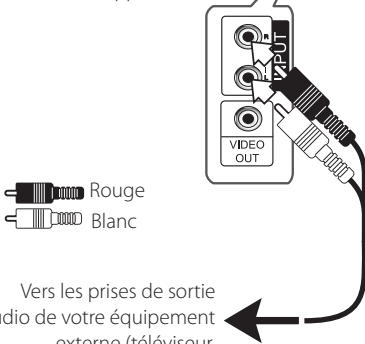
Arrière de l'appareil
