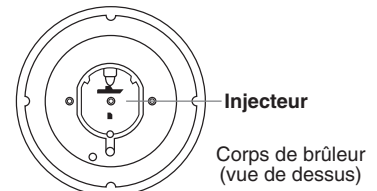
Brûleur de four - Injecteur four
