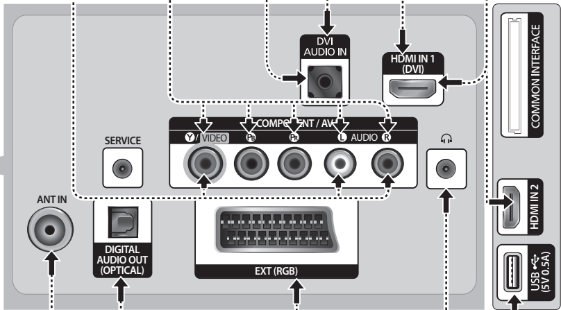
Panneau arrière du téléviseur
